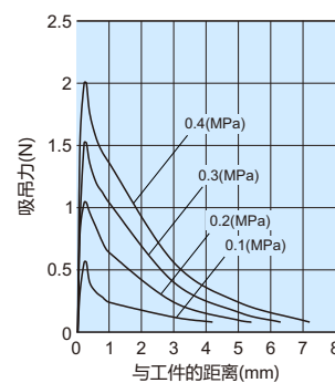
3A吸吊力和工件的距离
