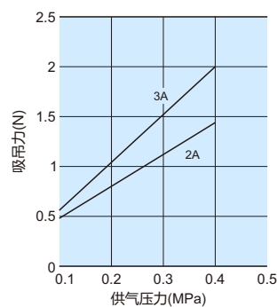
吸吊力
