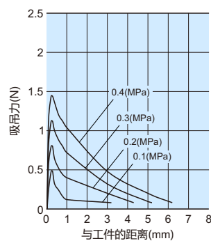
2A吸吊力和工件的距离
